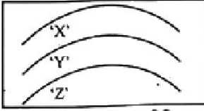
চিত্র: পৃথিবীর বায়ুমণ্ডলের বিভিন্ন স্তর
